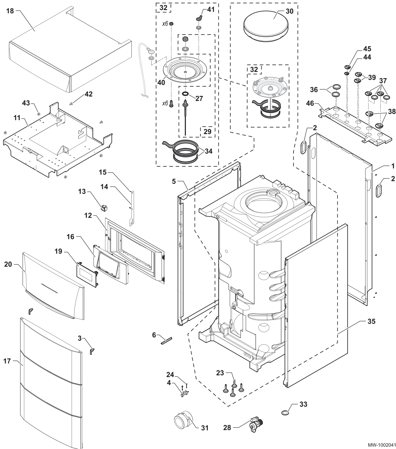
Afb.153 Basisframe
