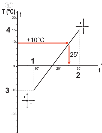
Afb.83 Tijdvertragingscurve voor starten back-up
