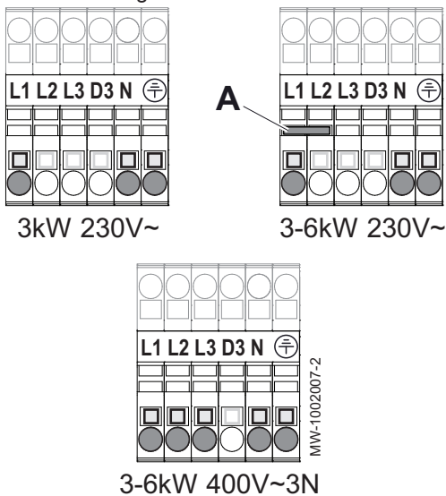
Afb.72 Configuraties
