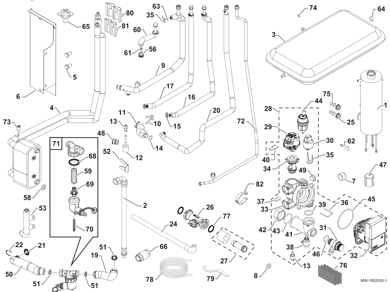
Afb.154 Hydraulisch circuit
