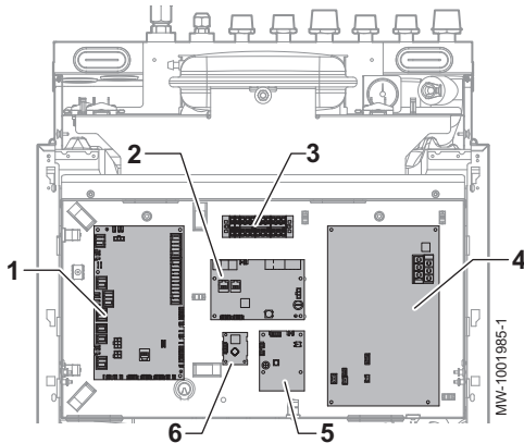
Afb.11 Plaats van de printen
