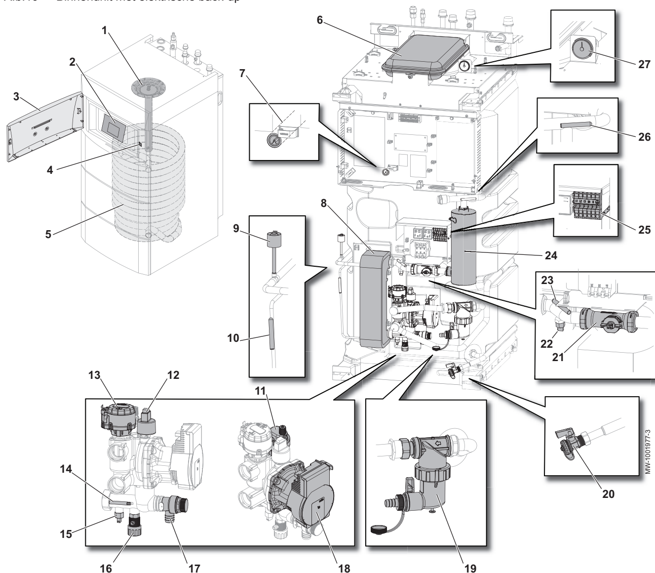
Afb.10 Binnenunit met elektrische back-up
