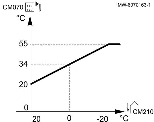
Afb.87 Verwarmingscurve met curve basis
