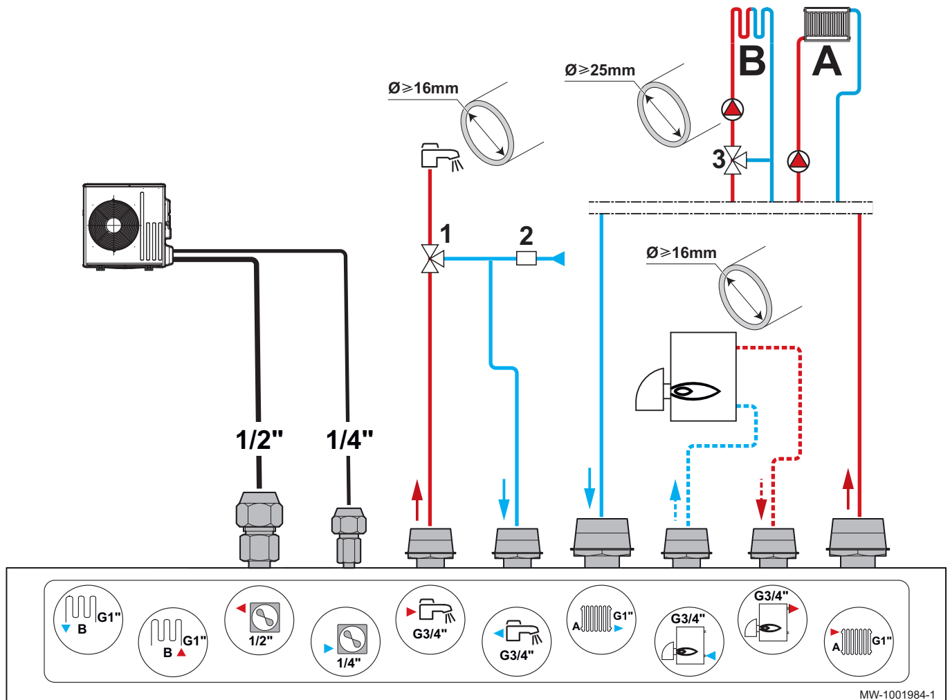
Afb.32 Mogelijke aansluitingen aan de binneneenheidszijde
