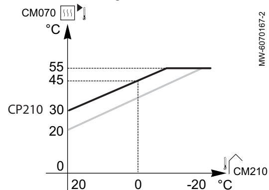
Afb.87 Verwarmingscurve met curve basis
