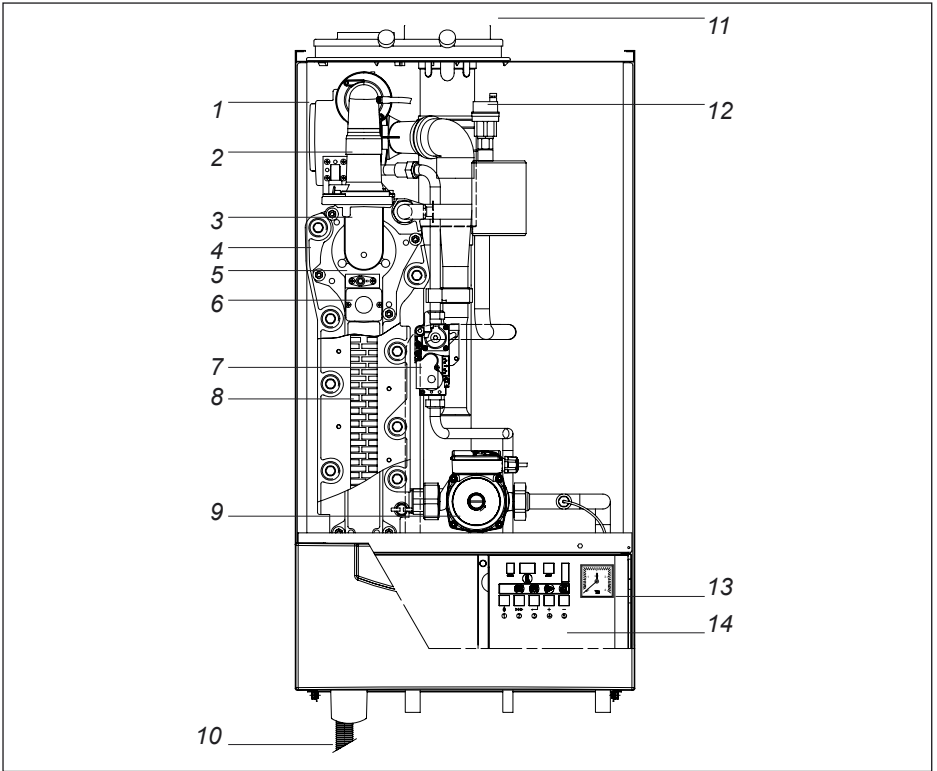
Afb. 02 Solotoestel 00.W3H.79.00053
